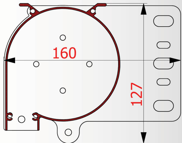
Staffa Speciale Tipo 2 per Posa In Nicchia: (disponibile su richiesta)
