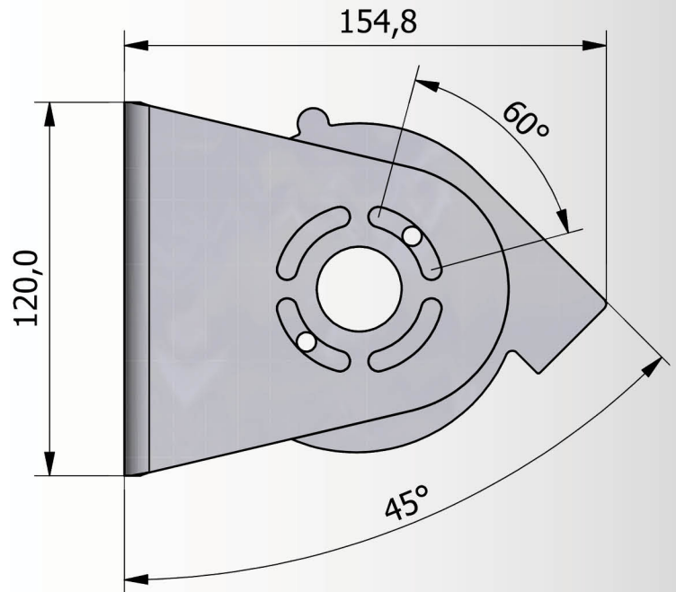
Staffa Speciale per posa CG Cass. a Parete: (disponibile su richiesta)
