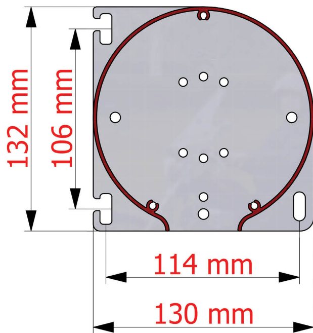
Installazione in Nicchia:
