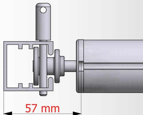
Posizione del Frontale nella Guida con Spine:
