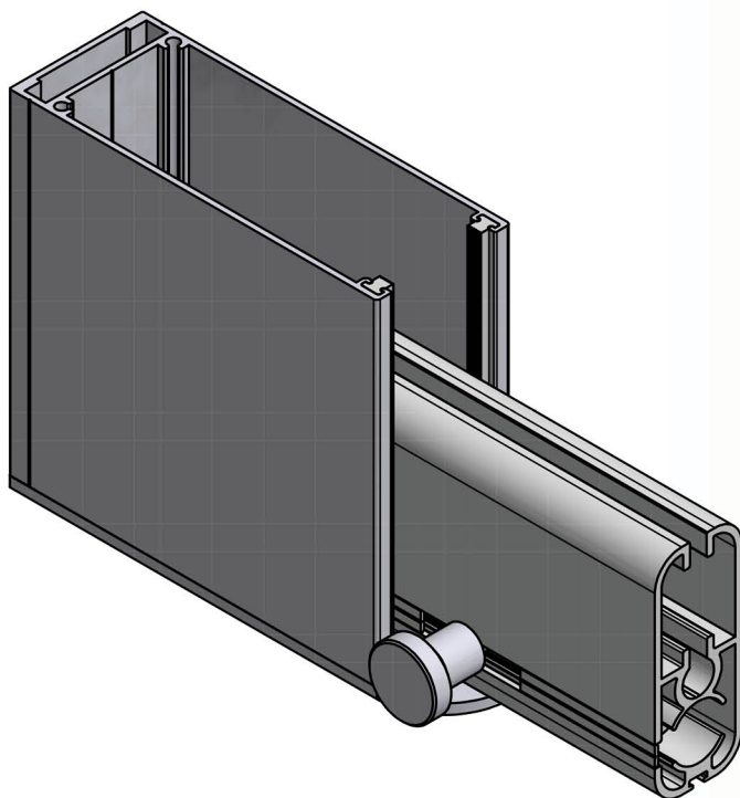
Optional Chiavistello Solo per Tende Manuali: Sezione del cassonetto, e posizione della doppia steccatura sul rullo avvolgitore: (da richiedere all'ordine)
