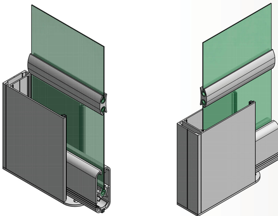
Sezione del frontale, fragitratta e telo nella guida:
