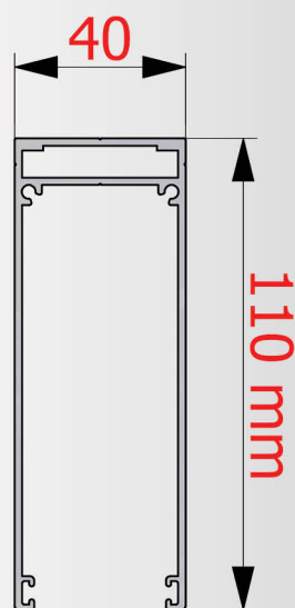
Sezione Guida 110 x 40:
