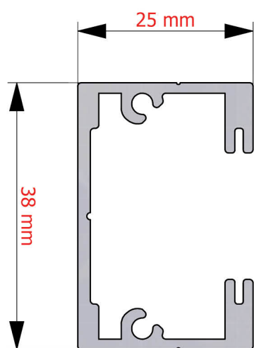
Sezione Profilo Guida:
