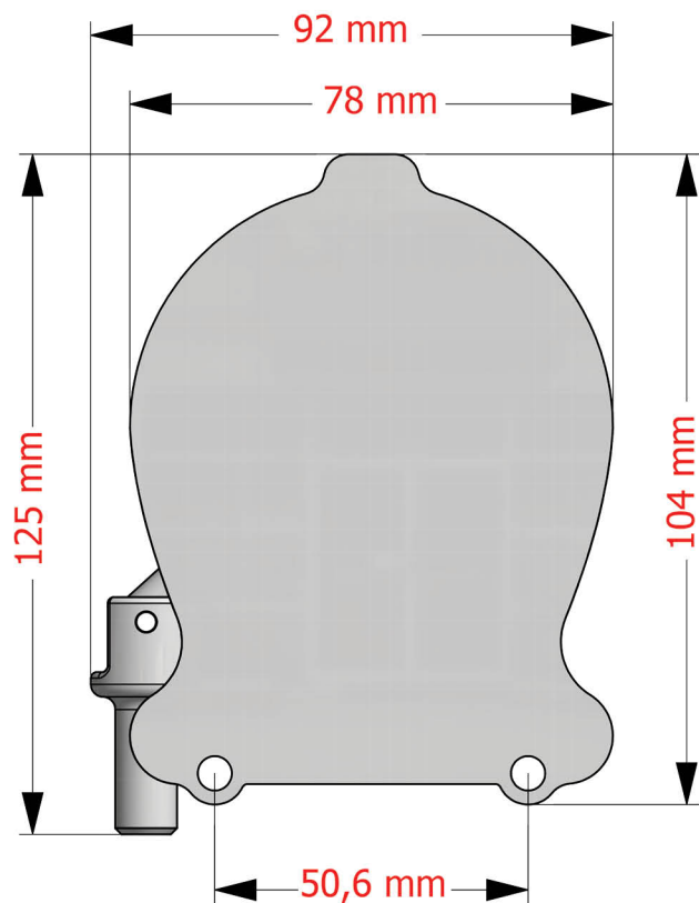
Vista laterale installazione a nicchia:
