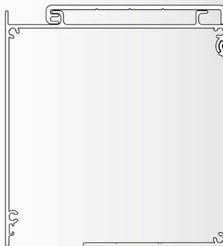
Vista laterale testata cassonetto:
