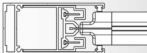
Sezione guida con sistema zip:
