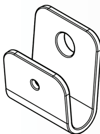
Staffa parete:
