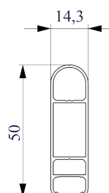
Ingombri profilo:
