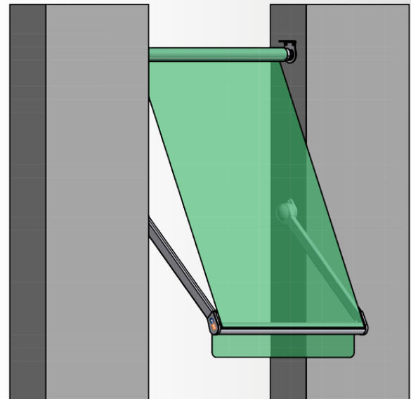
Installazione del rullo e del braccetto in nicchia: (standard)
