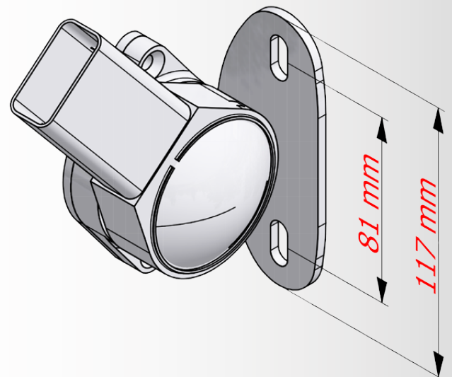
Staffa con Ingombri del braccetto per installazione in facciata:
