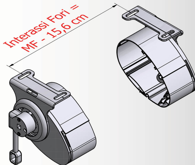
Modello ad Arganello
