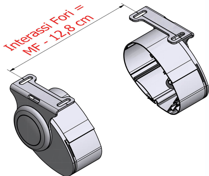
Modello a Motore
